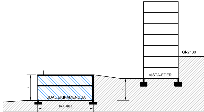
SECCION A-A'
