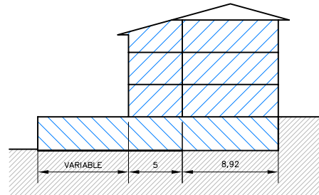
SECCION A-A'
