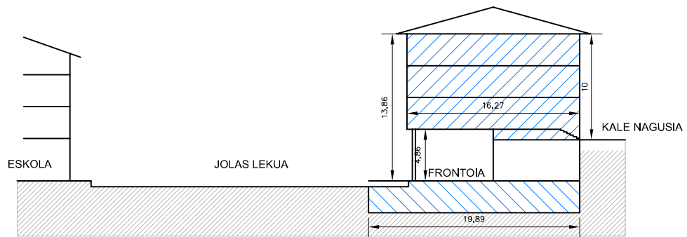
SECCION A-A'
